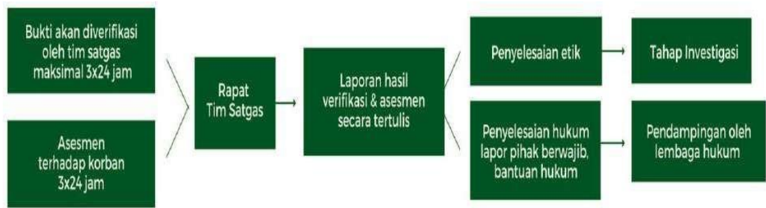
Gambar 5.4 Tahap Verifikasi
